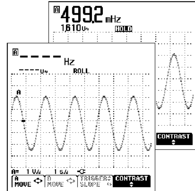
Рисунок 1-15. Запись осциллограмм в течение длительного периода времени
