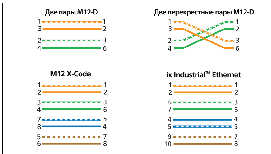
Рис. 12. Outlet Configurations - Промышленный Ethernet
