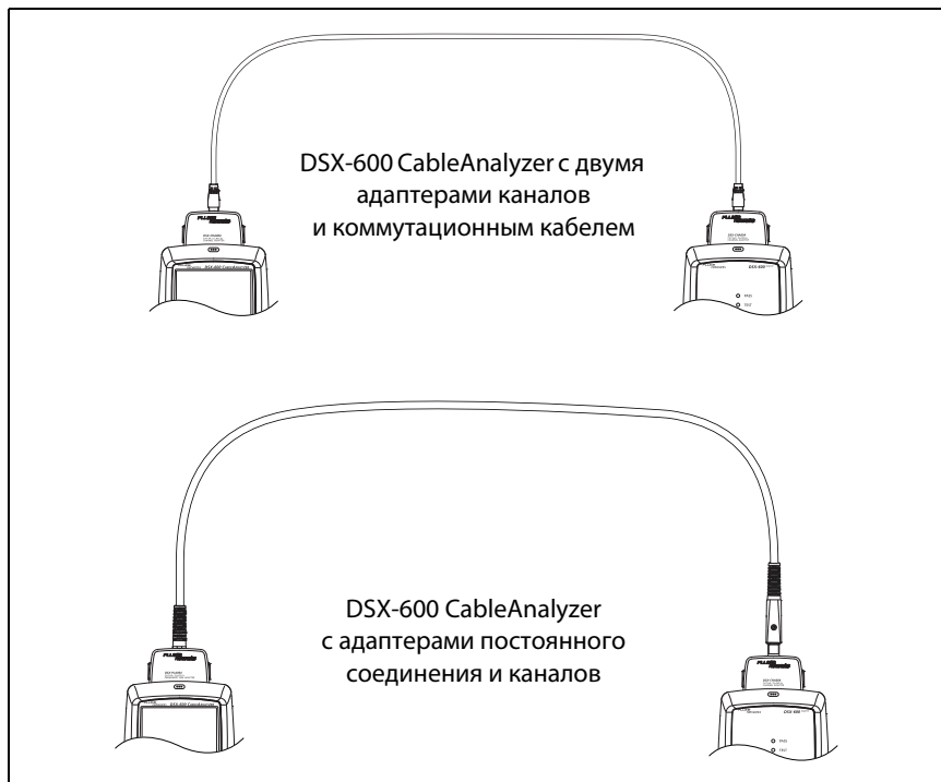
Рис. 6. Соединения для просмотра состояния батареи удаленного блока
