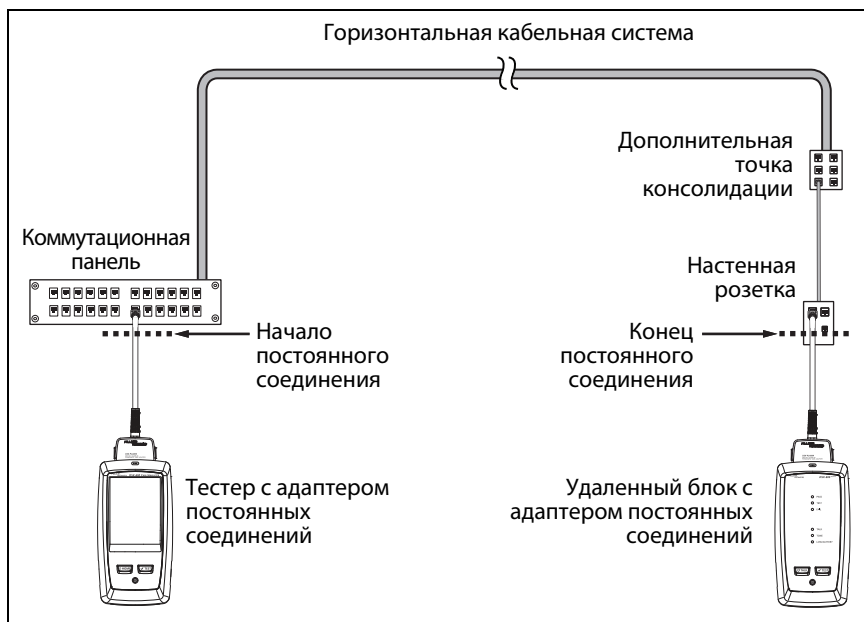
Рис. 14. Подключения постоянных соединений
