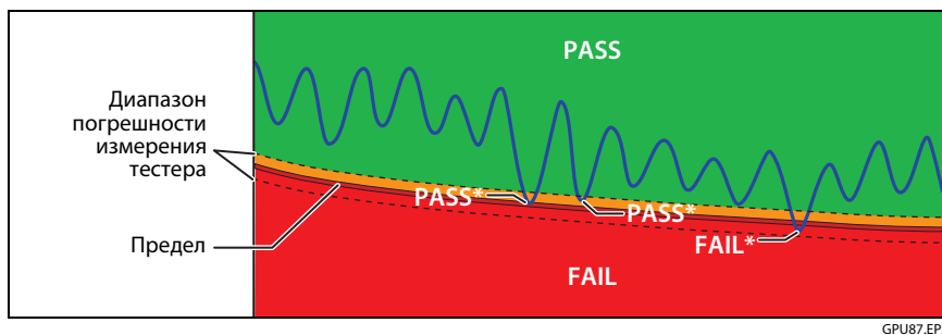
Рис. 16. Результаты «PASS*» и «FAIL*»
