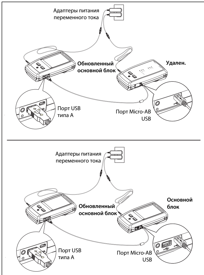
Рис. 33. Соединение блоков тестера для обновления программного обеспечения
